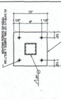
5) BASE PLATE DETAIL 1 1/2\"/>
