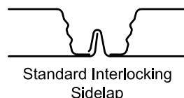
PLB-CD, PLB-CD AC, BCD or BCD AC FORMLOK
