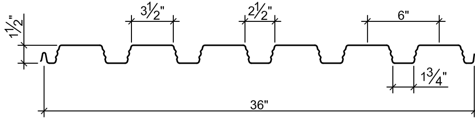
PLB or B FORMLOK
