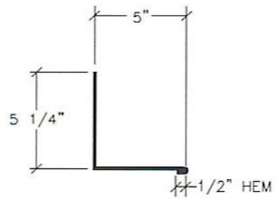
Sidewall (SW8)
