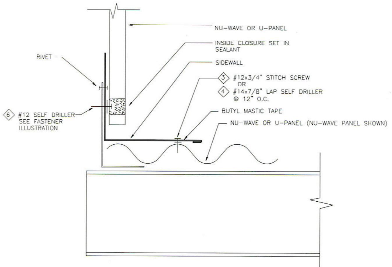
Sidewall (SW8)
