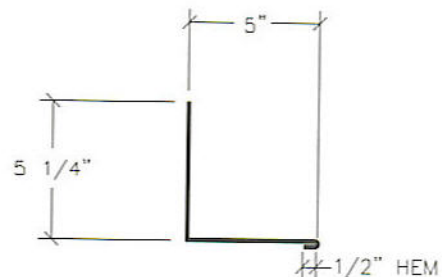
Sidewall (SW8)
