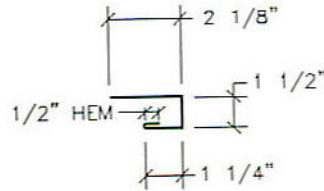
C-Metal (C12) Mini -V-Beam
